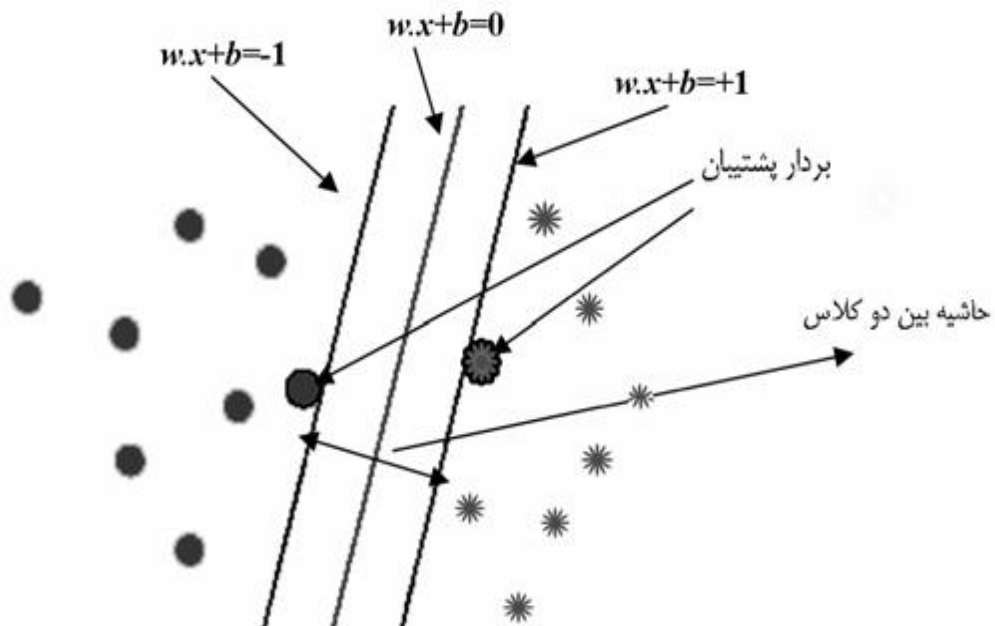
شکل ۱. روش حاشیه بیشینه جهت تعیین فرا صفحه بهینه، برای داده های قابل جداسازی
