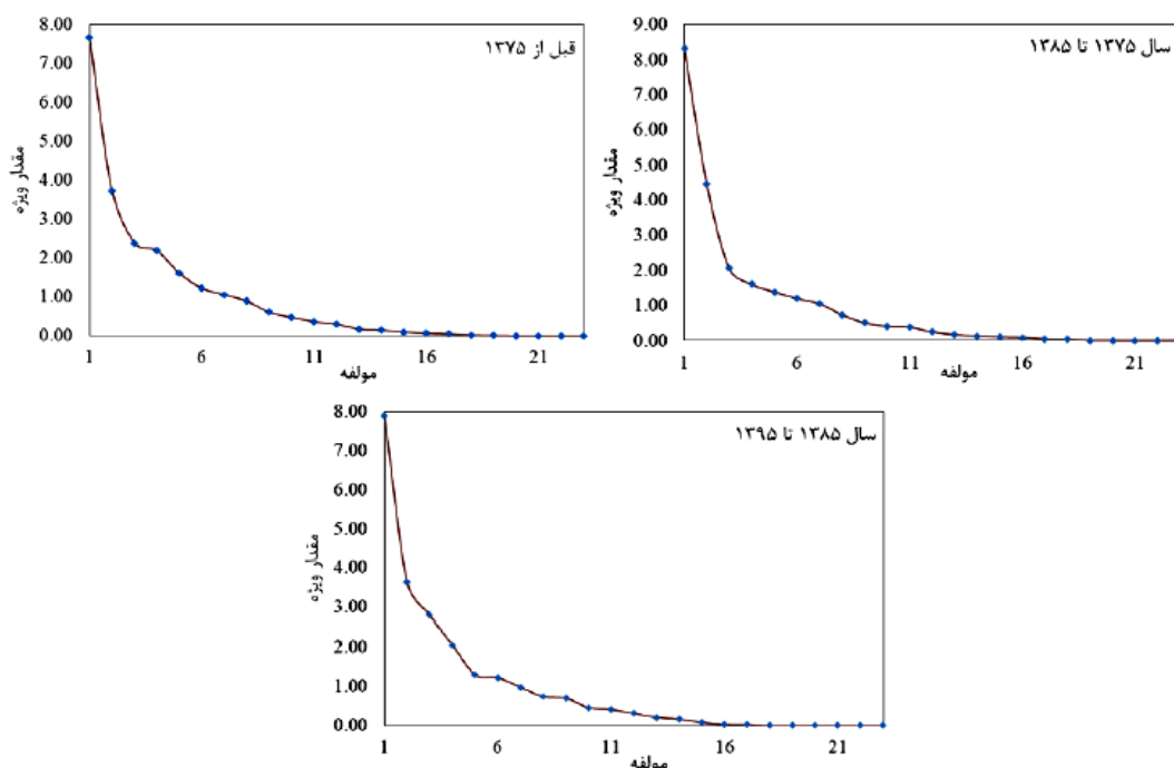
شکل ۲. نمودار سنگریزه برای تعیین مولفه‌ها در سه دوره مورد مطالعه
