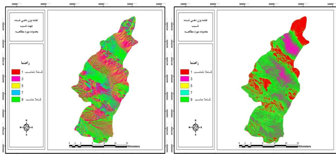
شکل ۵. وزن دار شده شیب (راست) و جهت شیب (چپ) محدوده مورد مطالعه
