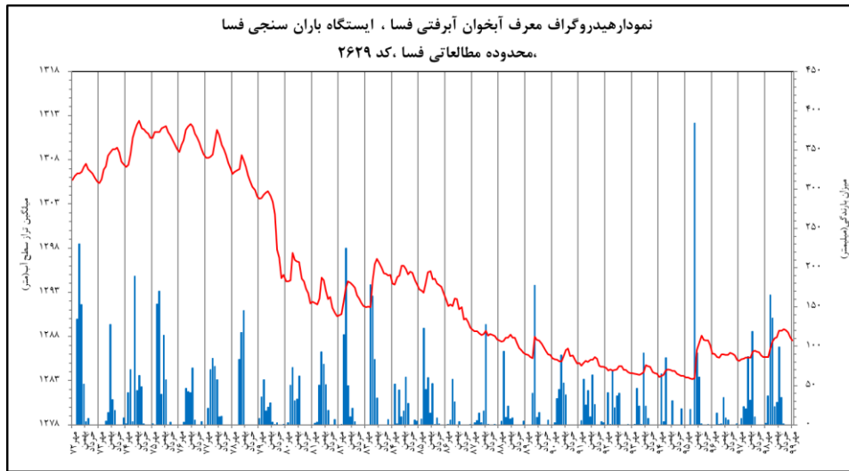
شکل ۵. تغییرات کلی چاه‌های دشت فسا از سال ۹۹-۷۲؛ برگرفته از: سازمان آب منطقه ای شهرستان فسا
