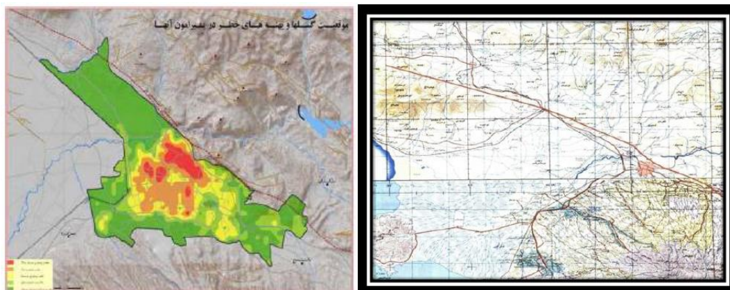
شکل ۲. موقعیت گسل‌ها و پهنه‌های خطر شهرستان تبریز (منبع: روستایی و همکاران، ۱۳۸۵)
